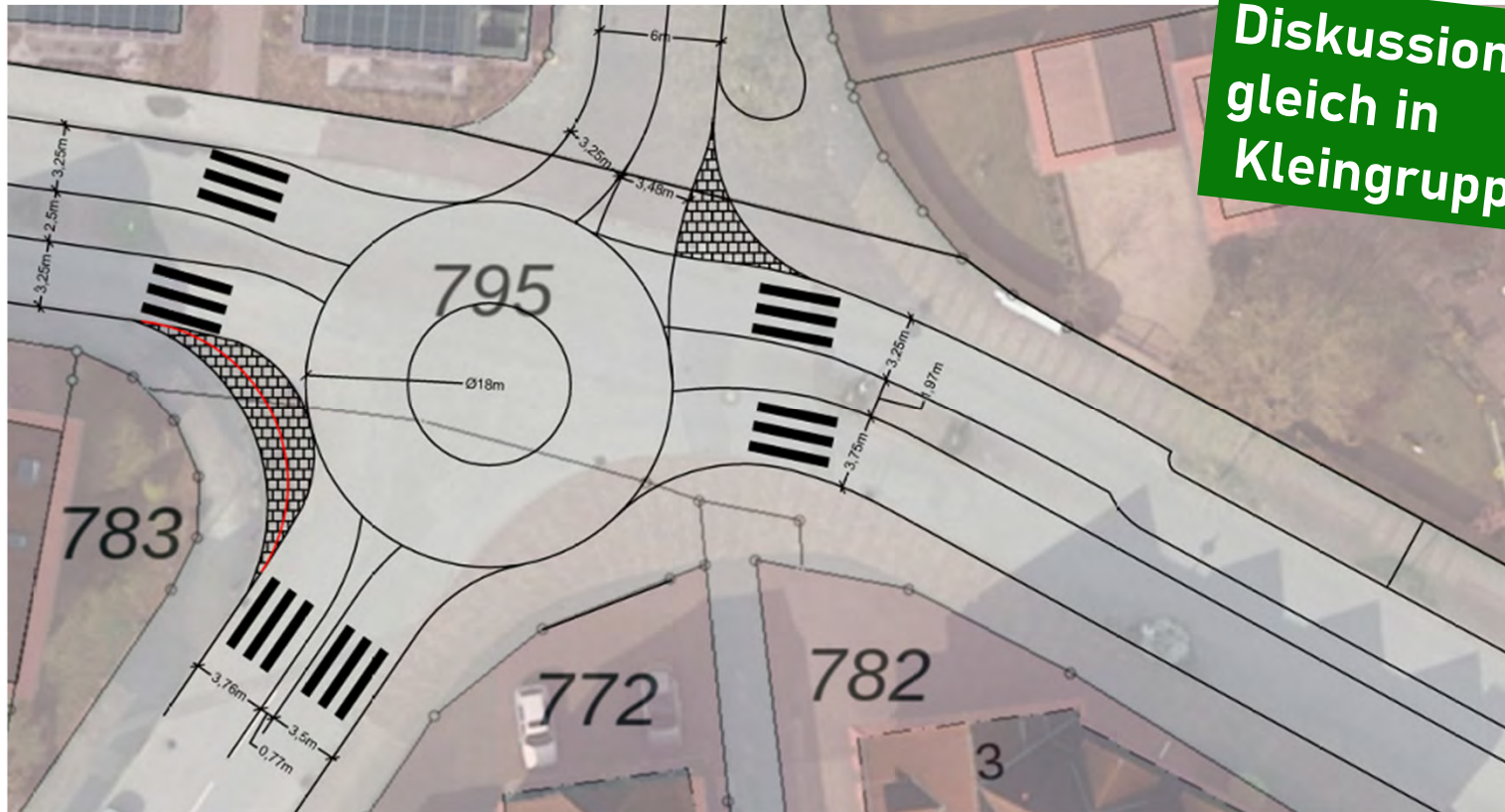
Vorentwurfsskizze: Knotenpunkt Rosenstraße / Lindenstraße / Parkstraße
